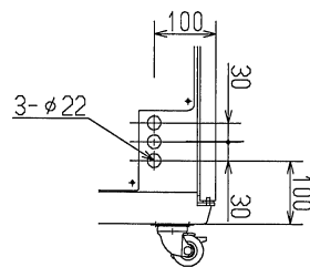
配線口詳細
